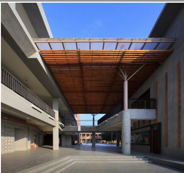
建築量體利用局部透空導入涼爽的西南風散熱。
